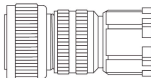
ACS3-CNPW5300 (для F180) Mil-Spec: MIL 3106A22-22S
