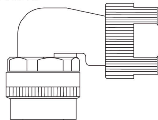
ACS3-CNPW6D00 (F100 ~ F180 с тормозом) Mil-Spec: CMV1-AP2S
