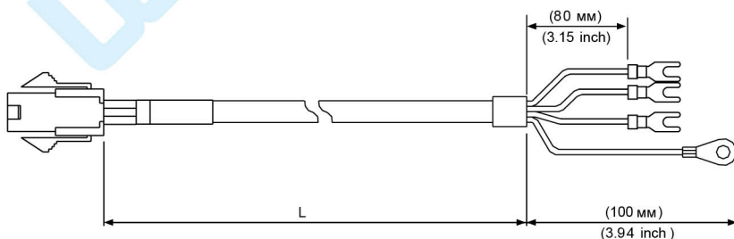
ACS3-CAPW3103, ACS3-CAPW3105, ACS3-CAPW3110, ACS3-CAPW3120, ACS3-CAPF3103, ACS3-CAPF3105, ACS3-CAPF3110, ACS3-CAPF3120 (для F80 и ниже)
