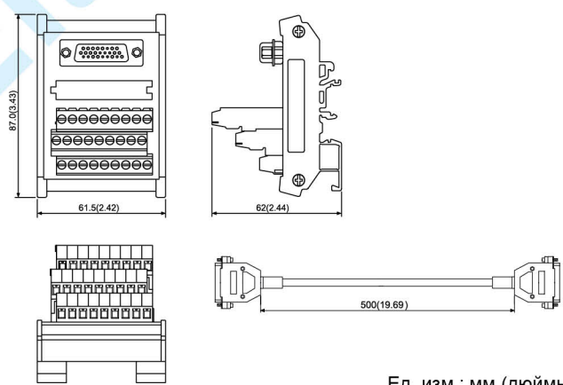
ACS3-MDTD2600 (для В3-M, F, E)
