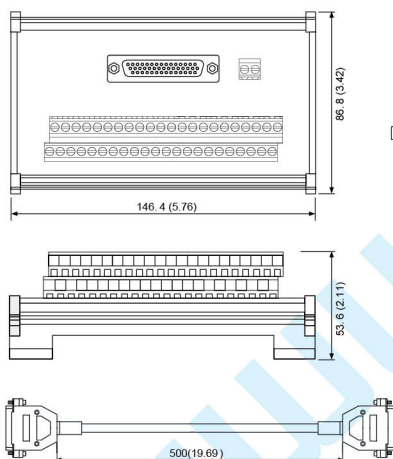
ACS3-MDTB4400 (для В3-L)
